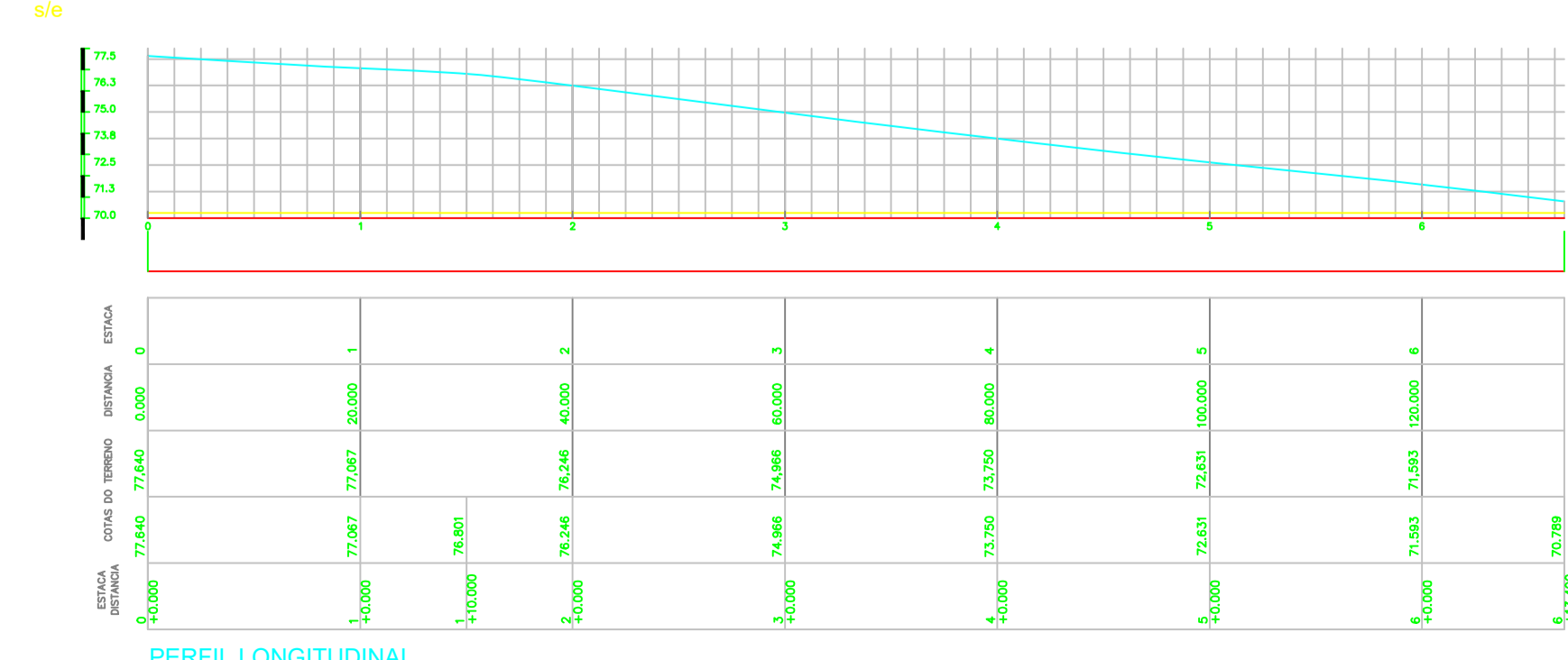
PERFIL LONGITUDINAL
