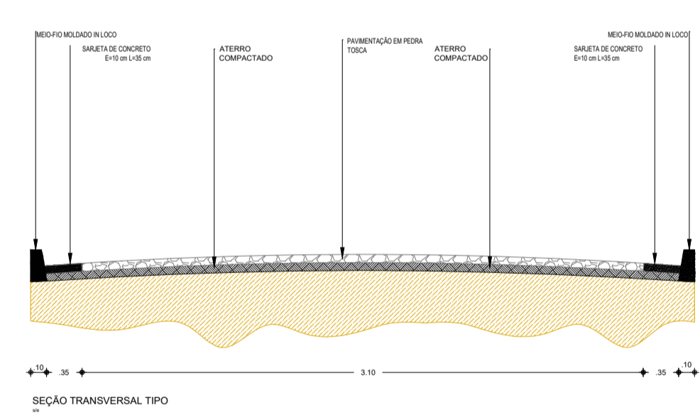
SEÇÃO TIPO - ESTACAS E0 A E3 TRECHO I
