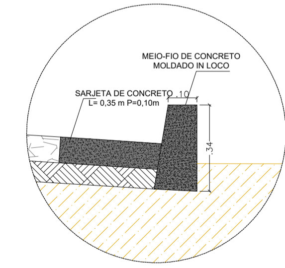
DETALHE SARJETA / MEIO FIO s/e
