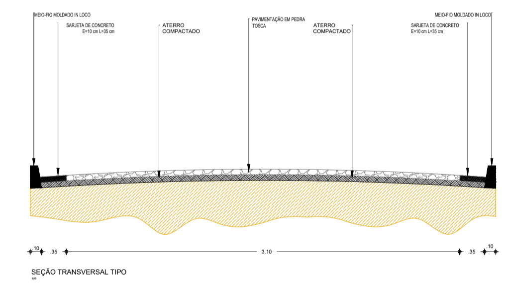
SEÇÃO TIPO - ESTACAS E4+12 A E7+17,79 TRECHO II
